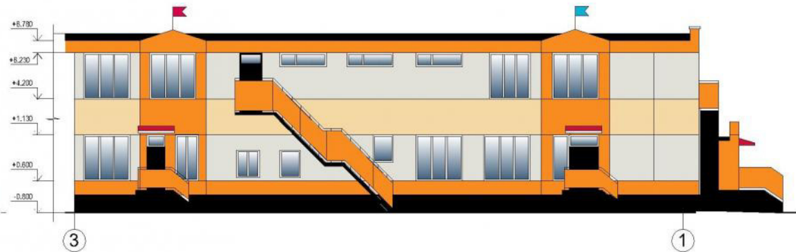
ФАСАД 1-3
