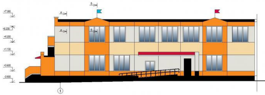
ФАСАД 1-2
